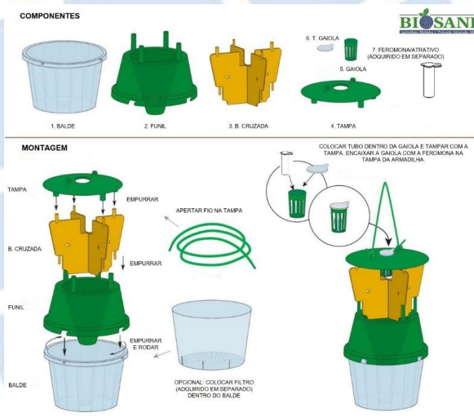
Figura 11.1 - Instruções de montagem do difusor na armadilha de funil com barreira cruzada. O tubo de polietileno (Fig. 10.1) deve ser instalado na vertical e com a tampa para cima no interior da gaiola.
